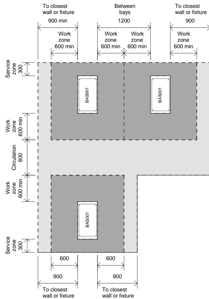
1 PLAN -STANDARD BASSINETS 1 : 50
