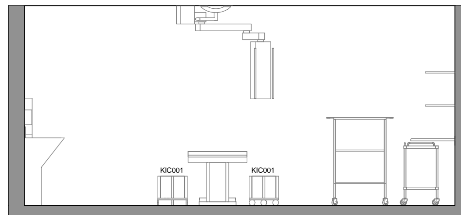
4 ELEVATION 1 : 50
