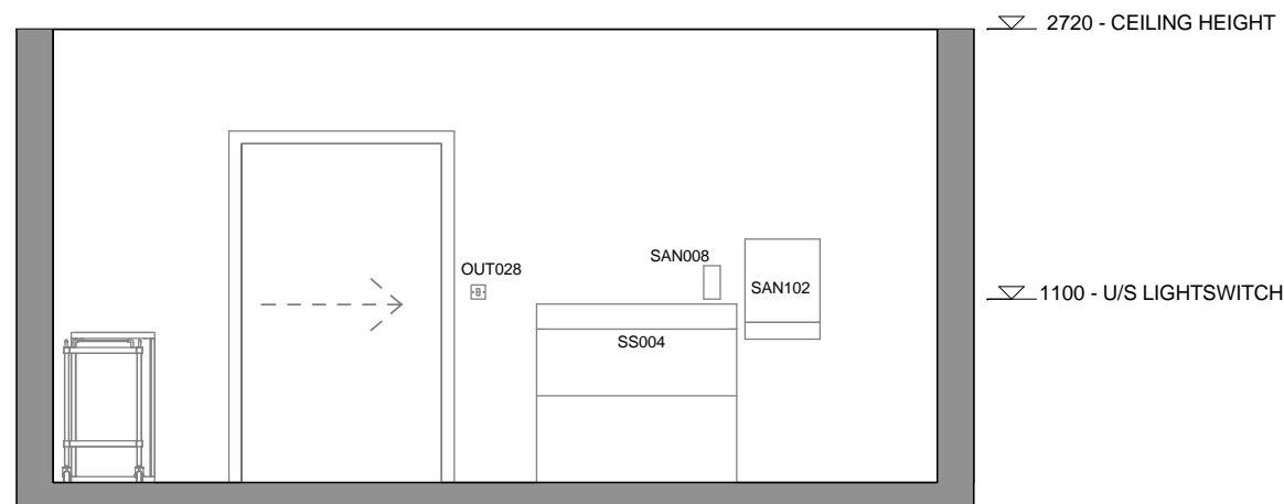
3 ELEVATION 1 : 50
